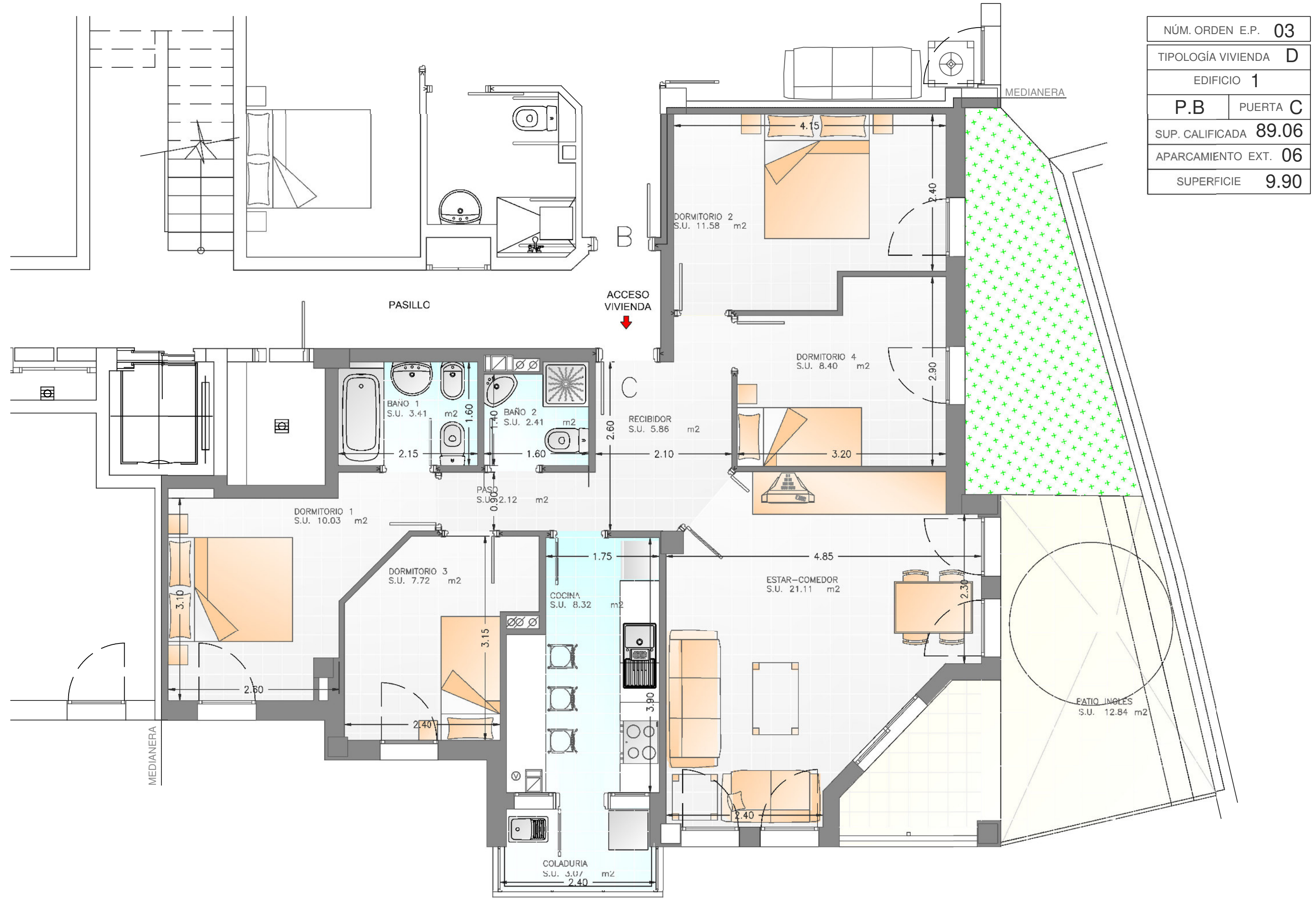
62 VIVIENDAS DE PROTECCIÓN PÚBLICA EN PEGUERA CALVIÀ - PLANTA BAJA - DISTRIBUCIÓN - E:1/50
