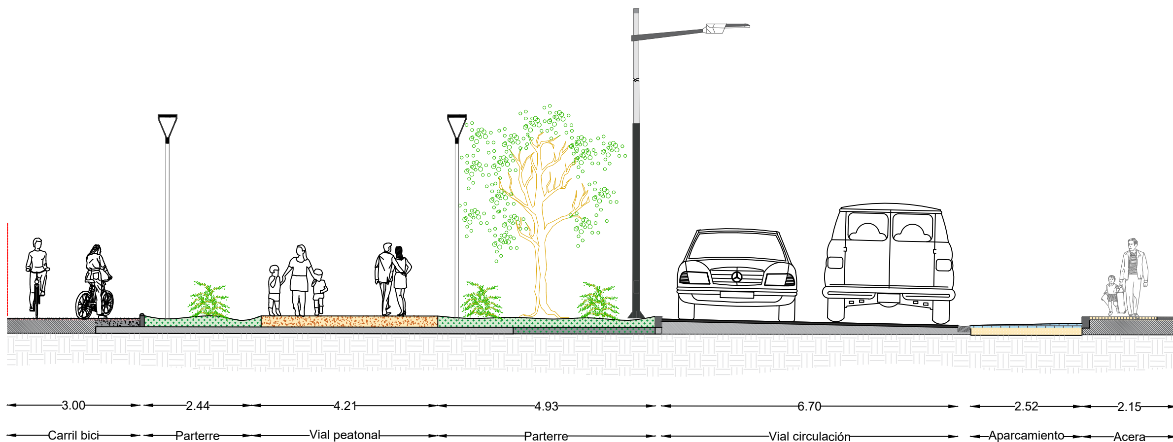
SECCIÓN B-B
