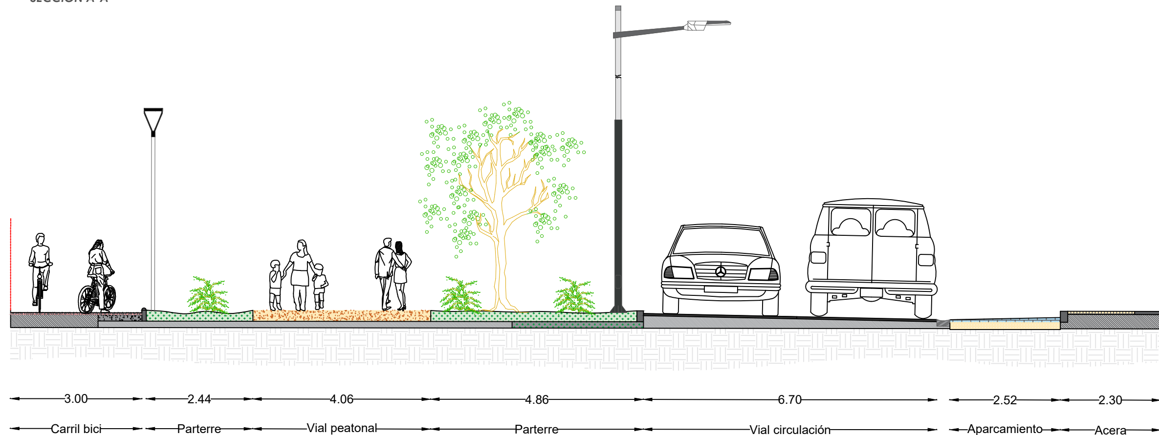
SECCIÓN A-A
